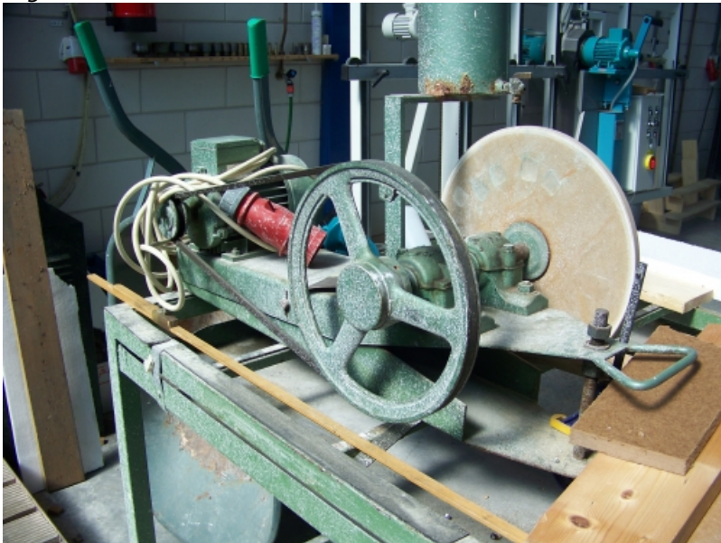
Niet afgeschermd draaiende delen
