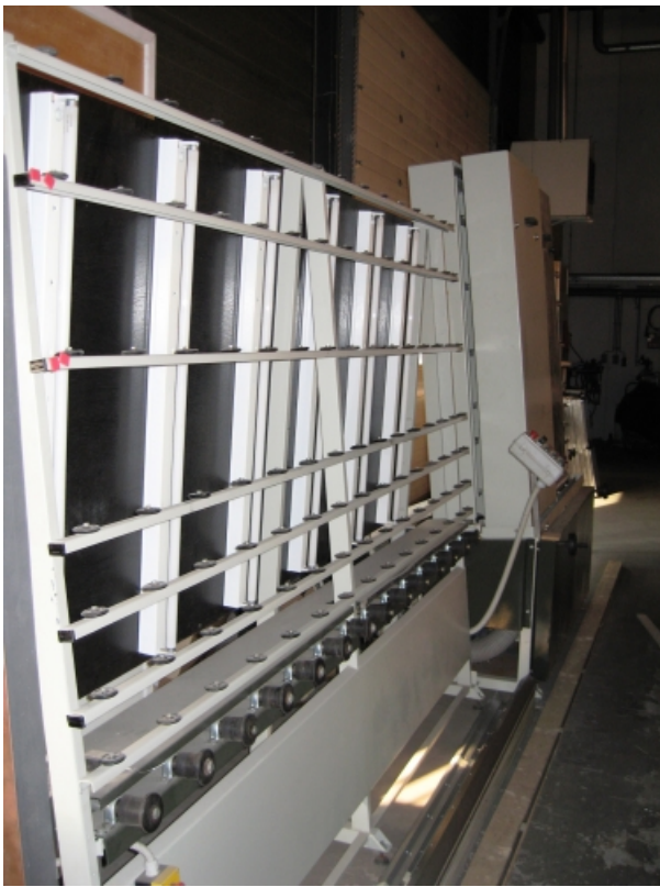
Verticale was- en schouwmachine
