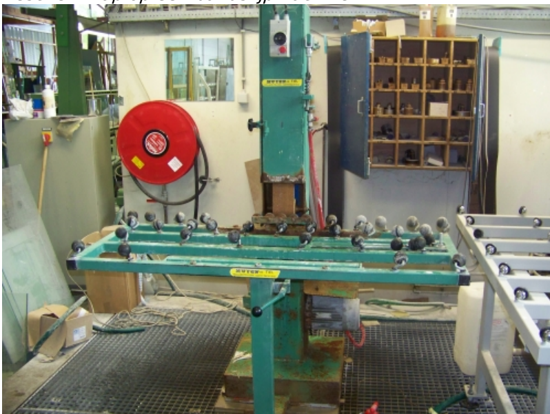
Bandslijpmachine zonder beschermkap
